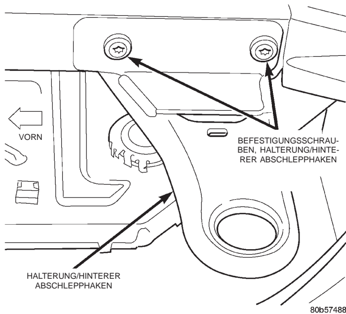
Abb. 4 Halterung des hinteren Abschlepphakens
