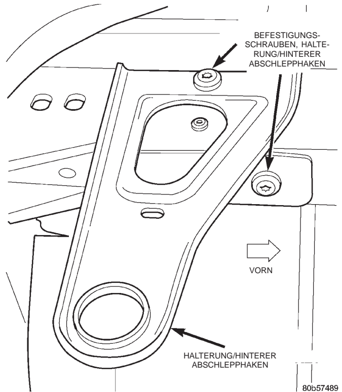
Abb. 5 Halterung des hinteren Abschlepphakens
