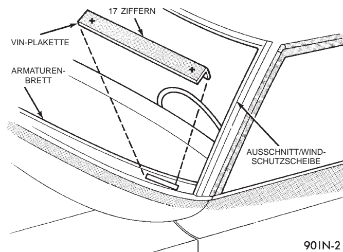
Abb. 2 Fahrgestellnummer (VIN-Plakette)
