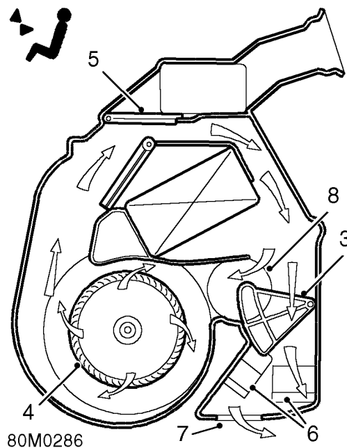
Fußraumbelüfter und Front- und Seitenscheibendefroster
