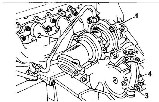
Bild 234 Befestigungsweise der Ölschmierleitung am Turbolader und Zylinderblock.
