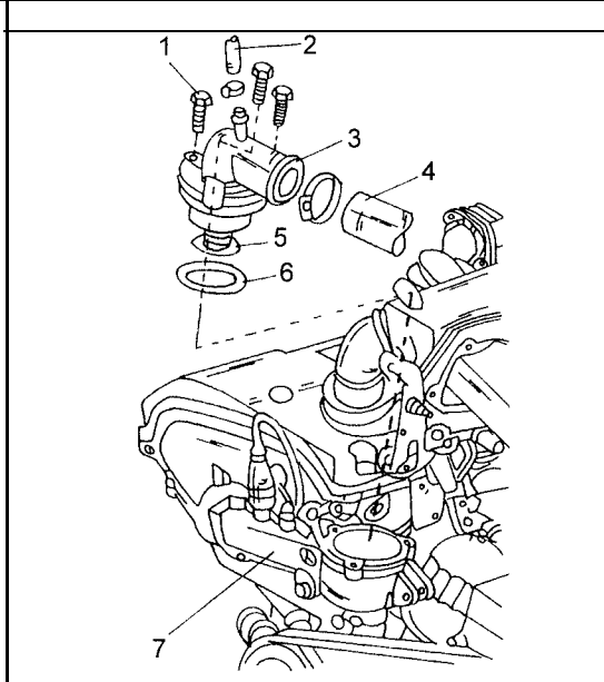
Bild 191 Einzelheiten zum Aus- und Einbau des Thermostats beim Benzinmotor. 1 Deckelschraube 2 Kühltittelschlauch zum Ausgleichsbehälter 3 Thermostatgehäusedeckel 4 Kühltittelschlauch zum Kühltiter 5 Thermostat 6 Dichtring 7 Thermostatgehäuse
