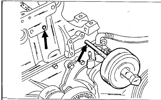
Bild 156 Die beiden Lagerbolzen an den Pfeilstellen aus dem Zylinderkopf herausziehen.
