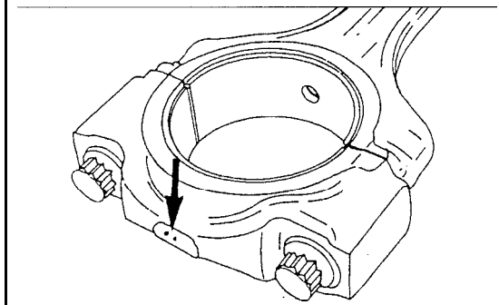
Bild 114 Die Kennzeichnung an der Unterseite der Pleuellagerstangen. Entweder ein oder zwei Körnerpunkte können eingeschlagen sein.
