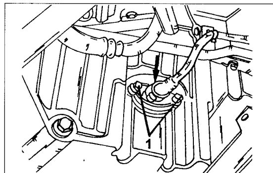
Bild 172 Die Lage des Ölstandanzeigers an der Seite der Ölwanne. Nach Lösen der Schrauben kann der Anzeiger herausgezogen werden.
