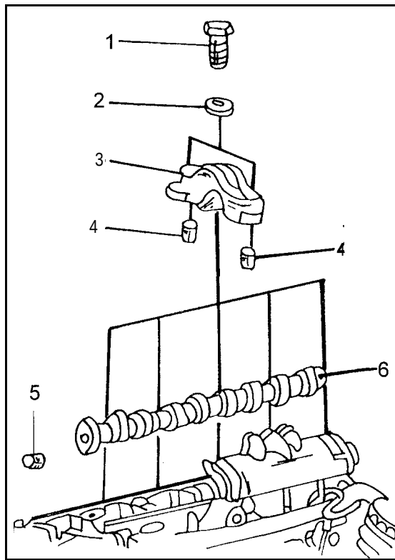
Bild 167 Einzelheiten zum Einbau der Nockenwelle. 1 Lagerdeckelschraube, 23 Nm 2 Unterlegscheibe 3 Nockenwellenlagerdeckel 4 Passhülsen 5 Passstift für Nockenwellenrad 6 Nockenwelle
