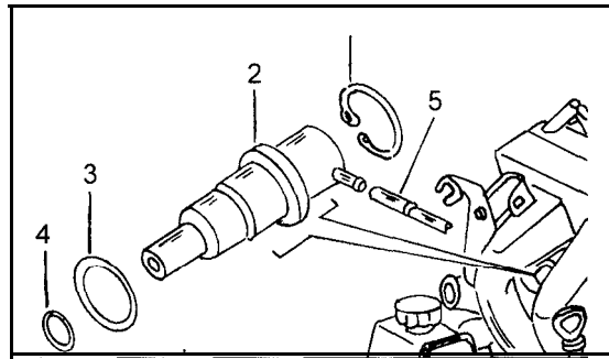
Bild 208 Die Lage des Kraftstoffdruckreglers am Motor.
