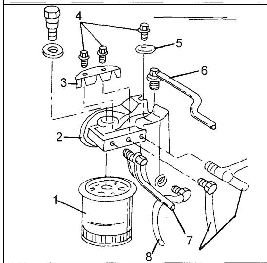
Bild 230 Einzelheiten zum Aus- und Einbau des Kraftstofffilters.
