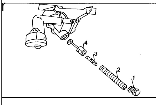
Bild 175 Die Teile des Überdruckventils der Ölpumpe. 1 Verschlussstopfen (50 Nm) 2 Druckfeder 3 Führungsstift 4 Kolben mit zwei Flächen
