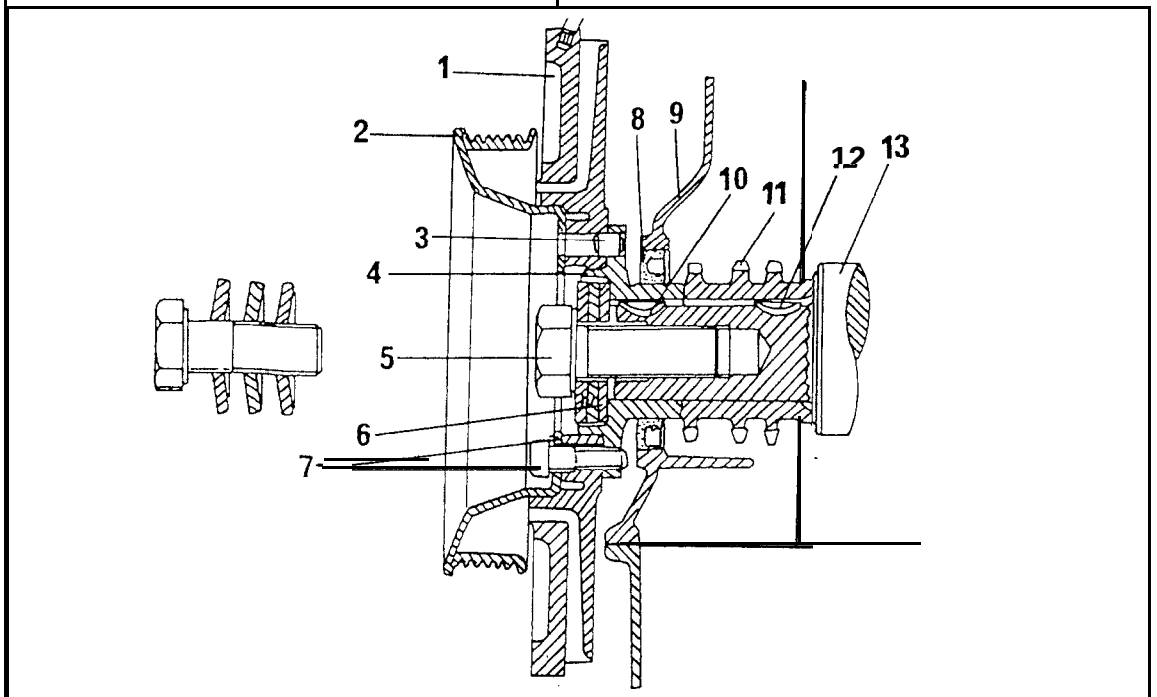
Bild 148 Schnitt durch die Vorderseite der Kurbelwelle. 1 Schwingungsdämpfer 2 Riemenscheibe 3 Passstift, 8 x 8 mm 4 Riemenscheibennabe 5 Schraube, M18 x 1,5 6 Federscheiben 7 Schrauben, M8 x 25 und Scheibe 8 Radialdichtring 9 Steuergehäusedeckel 10 Scheibenfeder(Keil) 11 Kurbelwellensterrad 12 Scheibenfeder 13 Kurbelwelle
