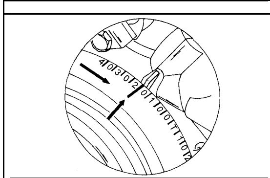
Bild 25 Die Kurbelwelle durchdrehen, bis der Zapfen an der Stirnseite des Motors gegenüber der langen Linie in der Gradeinteilung steht.
