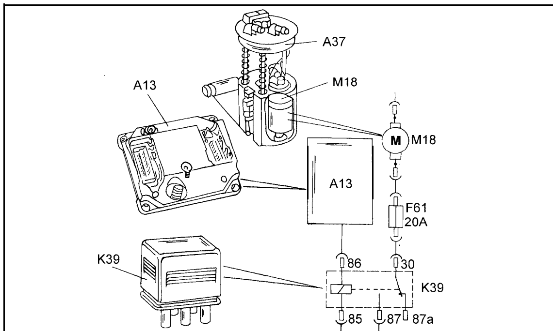
Bild 206 Der elektrische Stromverlauf zwischen Kraftstoffpumpe und Kraftstoffpumpenrelais. Die Kennzeichnungen sind im Text erwähnt. Die Zahlen unten rechts weisen auf die Bezeichnungen der Kabelanschlüsse.
