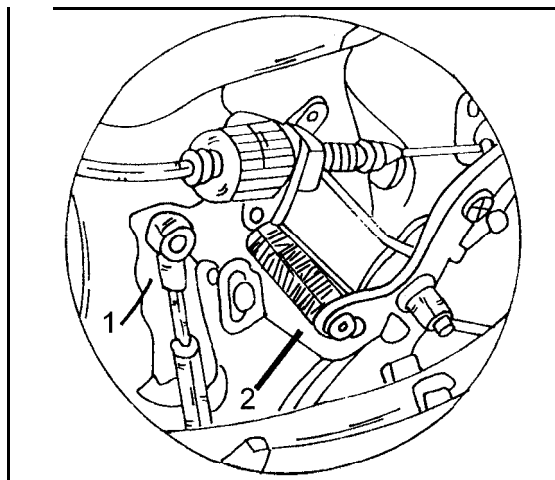
Bild 213 Verbindung des Gestänges (1) am Regelhebel (2) trennen, um die Gasbetätigung abzuschliessen.
