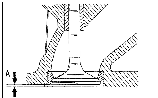
Bild 103 Das Mass „A“ muss beim Einziehen von neuen Ventilsitzringen und bei Verwendung von neuen Ventilen dem im Text angegebenen Wert entsprechen.
