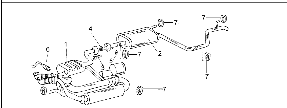
Bild 351 Die Auspuffanlage bei eingebautem Benzinmotor. 1 Vordere Auspuffanlage 2 Hintere Auspuffanlage 3 Flanschschrauben 35 - 30 Nm 4 Dichtung 5 Mutter 6 Lambda-Sonde 7 Aufhängungsgummischlaufen
