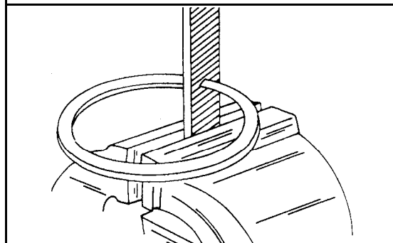
Bild 68 Vergrössern eines Pleu- ellenagerstossspiels.
