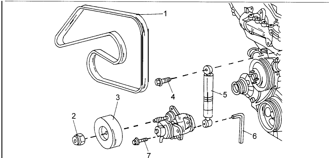
Bild 190 Einzelheiten der Befestigung des Spanndämpfers. 1 Polyriemen 2 Sundmutter 3 Spannrolle 4 Kombischraube 5 Spanndämpfer 6 Inbusschlüssel (zum Gegenhalten) 7 Kombischraube
