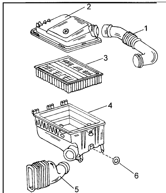
Bild 211 Die Einzelteile des Luftfilters. 1 Ansaugluftschlauch 2 Luftfilterdeckel (Oberteil) 3 Luftfiltereinsatz 4 Luftfiltergehäuse 5 Anschlussstutzen zum Luftfilter 6 Befestigungsring
