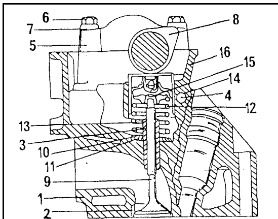
Bild 101 Schnitt durch den Zylinderkopf mit einem Auslassventil.
