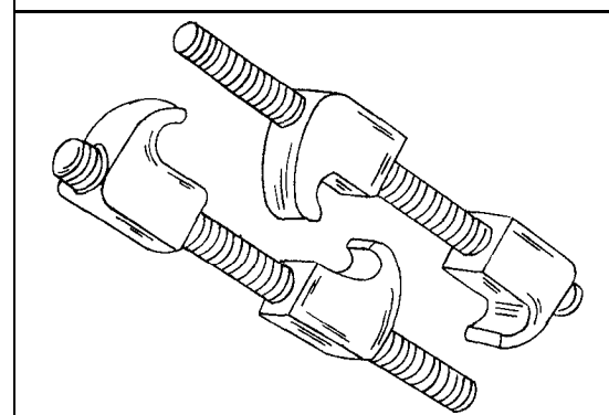
Bild 282 Federspannhaken dieser Form eignen sich gut zum Zusammenspannen der Hinterfedern. Aufgrund der hohen Spannung der Federn müssen sie natürlich kräftig genug sein.
