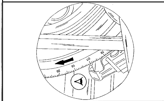
Bild 161 Grossansicht der Gradkennzeichnungen am Schwingungsdämpfer der Kurbelwelle. Die Kurbelwelle in Pfeilrichtung durchdrehen, bis die OT-Stellung erhalten wird.
