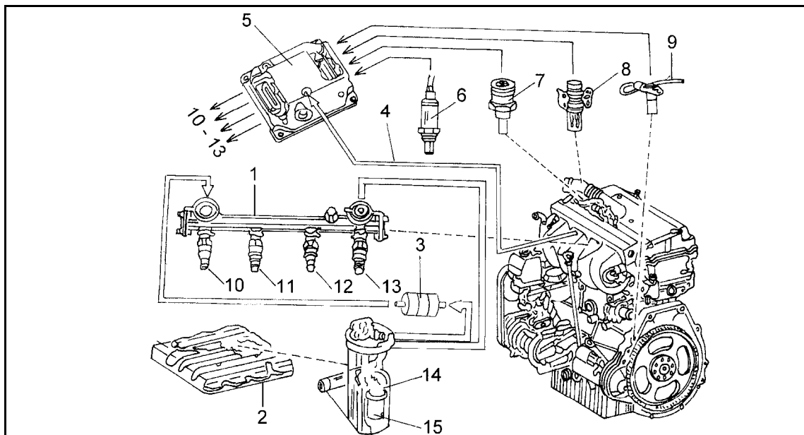
Bild 201 Die Teile der PMS-Kraftstoffeinspritzung. 1 Kraftstoffverteilerrohr 2 Kraftstofftank 3 Kraftstofffilter 4 Ansaugrohrdruck 5 Elektronisches Steuergerät 6 Beheizte Lambda-Sonde 7 Temperaturgeber 8 Ansaugrohr-Temperaturgeber 9 Drehzahlgeber der Kurbelwelle 10 Einspritzventil 11 Einspritzventil 12 Einspritzventil 13 Einspritzventil 14 Tankgeber 15 Kraftstoffpumpe
