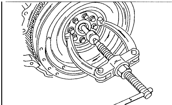
Bild 146 Beim Ausziehen des Kugellagers der Kurbelwelle muss das Schwungrad angeschraubt sein.
