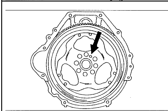
Bild 147 Die Fluchtbohrung der Antriebsscheibe befindet sich an der gezeigten Stelle.
