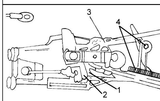
Bild 327 Anschlussweise der Bremsseile am Ausgleich des Feststellbremsseils. 1 Ausgleichshebel 2 Schraube, Bremsseil an Ausgleichshebel, 18 Nm 3 Einstellschraube 4 Rückzugfeder
