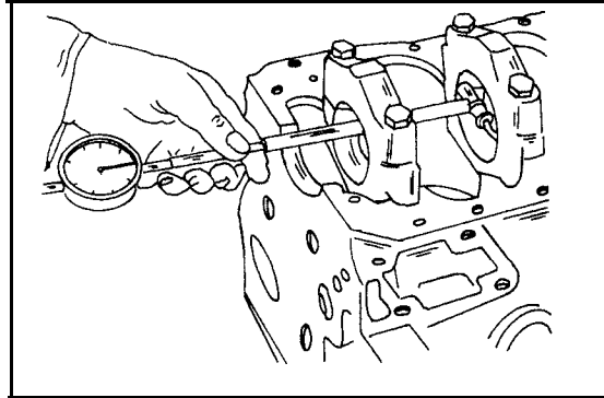
Bild 78 Ausmessen der Hauptlagerdurchmesser mit einer Innenmessuhr.
