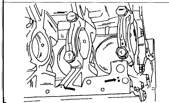
Bild 137 Die Pfeile weisen auf die Körnerschläge zur Kennzeichnung der Pleuellagerbohrungstoleranzen. Lagerschalen sind entsprechend der Kennzeichnung zu verwenden.
