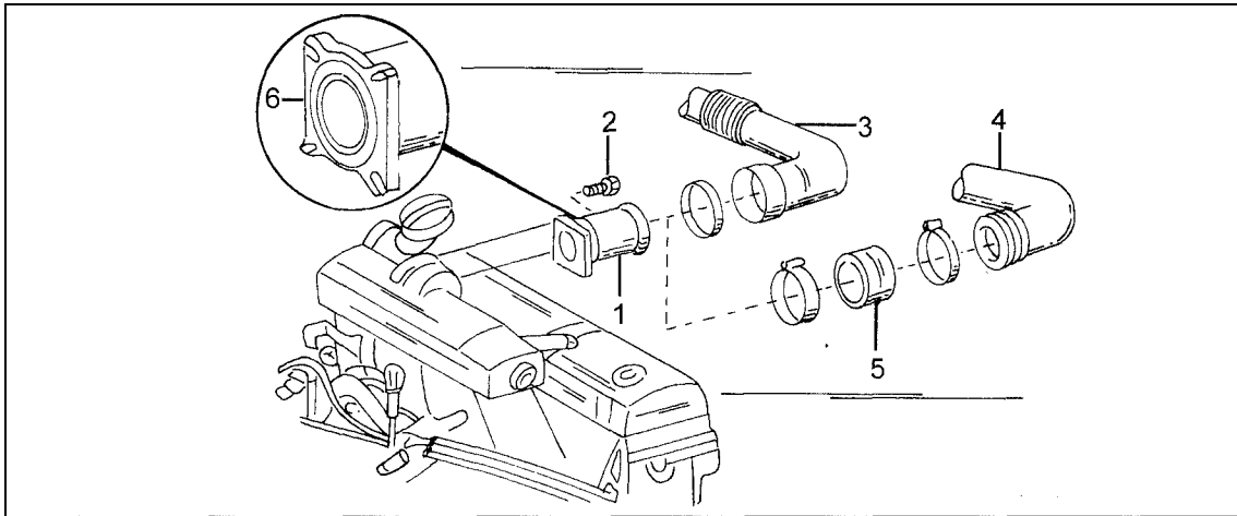
Bild 229 Zum Aus- und Einbau der Mischkammer.
