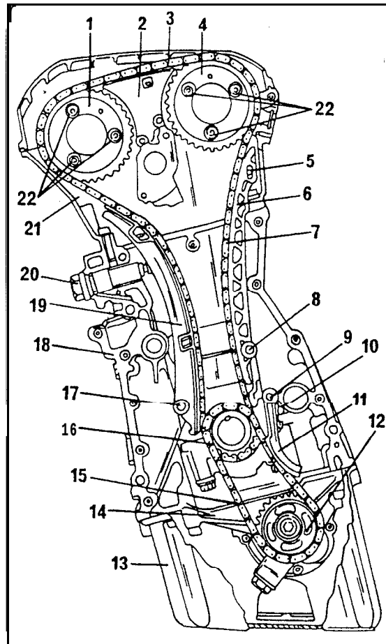
Bild 47 Verlegung der Steuerkette und Kette des Ölpumpenantriebs.
