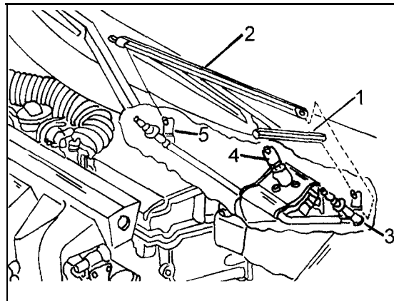
Bild 348 Einzelheiten zum Aus- und Einbau des Wischergestänges.
