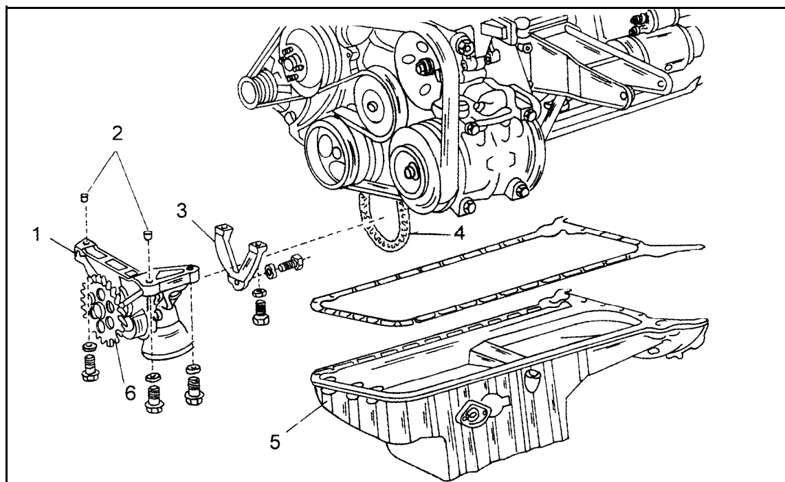
Bild 173 Befestigungsweise der Ölpumpe und Ölwanne am Motor. 1 Ölpumpe 2 Passhülsen 3 Verstärkungswinkel 4 Ölpumpenkette 5 Ölwanne 6 Antriebskettenrad der Ölpumpe
