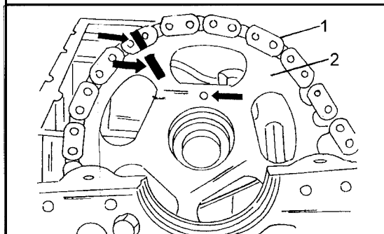
Bild 162 Kennzeichnung des Steuerrades der Nockenwelle (Pfeile links) und der Passstiftes des Steuerrades (Pfeil in der Mitte). 1 Steuerkette 2 Steuerrad
