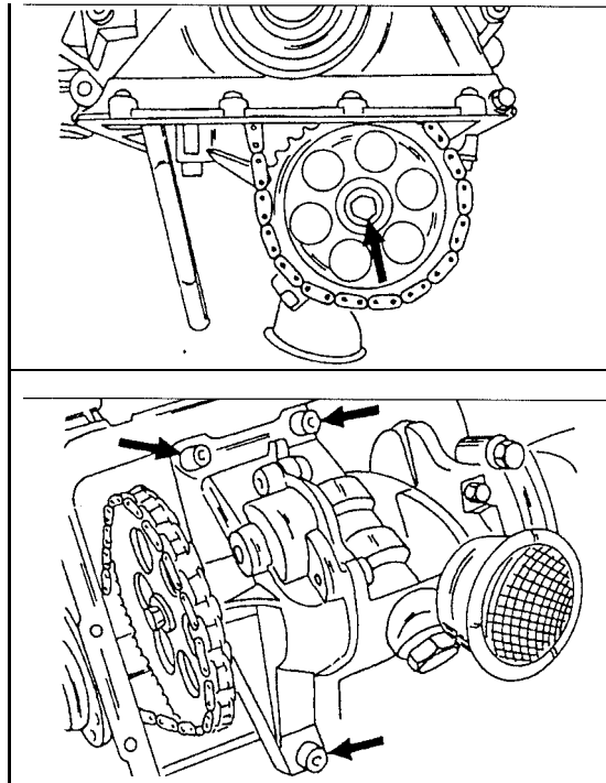
Bild 179 Die Schraube (Pfeil) in der Mitte des Ölpumpenkettenrades lösen und das Rad zusammen mit der Kette abziehen.
