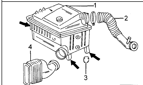
Bild 231 Einzelheiten um Aus- und Einbau des Luftfilters.
