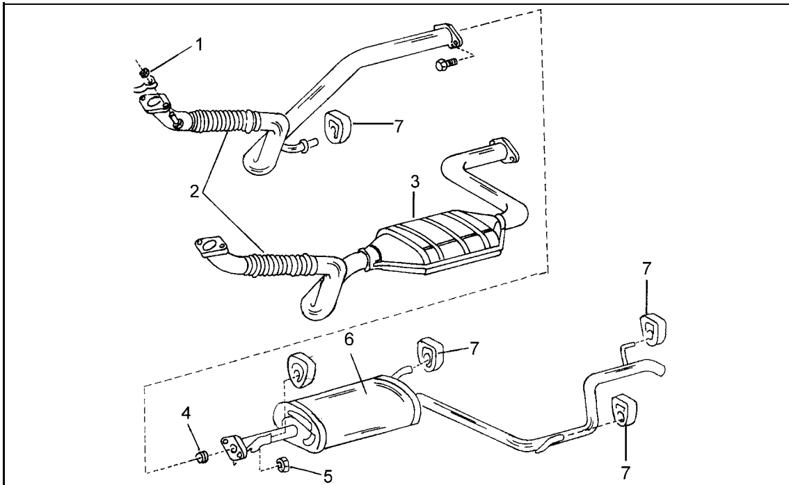
Bild 350 Die Auspuffanlage bei eingebautem Dieselmotor. 1 Selbstsichernde Mutter 2 Vordere Auspuffanlage, je nach Ausführung mit oder ohne Katalysator 3 Oxidationskatalysator 4 Dichtung 5 Selbstsichernde Mutter 6 Hintere Auspuffanlage 7 Aufhängungsgummischlaufen
