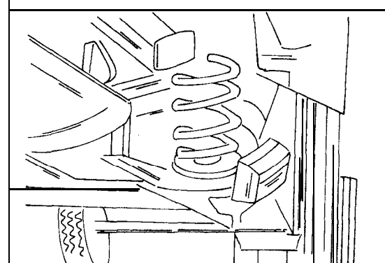
Bild 281 Nach Abschrauben des Hinterrades wird man die Hinterfeder zwischen dem Schwingarm und dem oberen Federsitz sehen.
