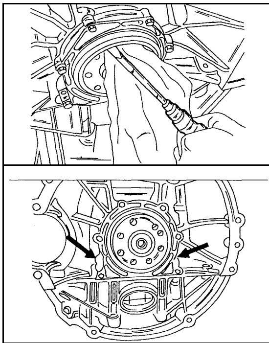
Bild 149 Aushebeln des hinteren Kurbelwellendichtringes. Den Lappen an der gezeigten Stelle unterlegen.
