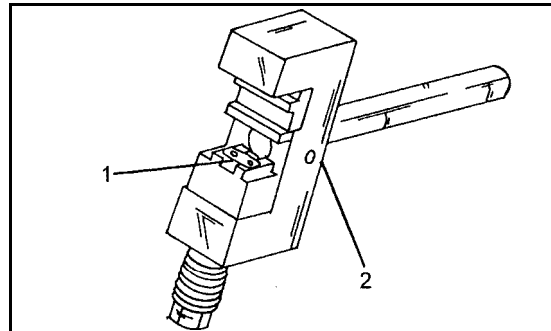
Bild 57 Montagewerkzeug für die Befestigung eines Kettenglieds an der neuen Steuerkette. 1 Verbindungsschraube 2 Montagewerkzeug
