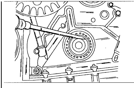
Bild 151 Aushebeln des vorderen Dichtringes aus dem ein- gebauten Steuerdeckel.
