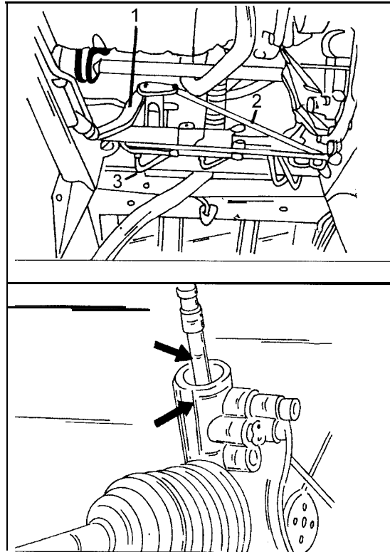
Bild 300 Einzelheiten zum Ausbau der Lenkung. Die beiden Versteifungen (1) und (2) von der Vorderachse abschrauben und die Ausgleichsleitung (3) an der Unterseite abschliessen.
