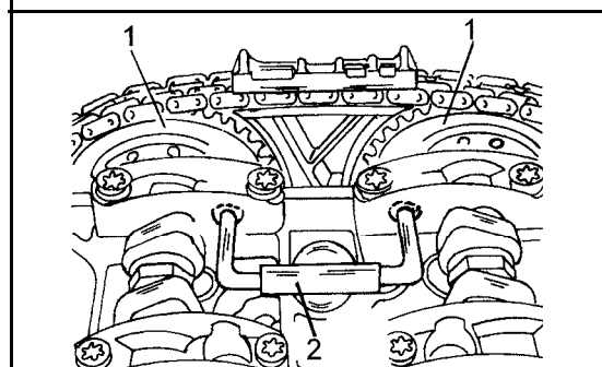
Bild 60 Die beiden Nockenwellenstößel werden durch Einschieben der Arretierbolzen in der richtigen Stellung gesperrt. Dies verhindert, dass die Pleuel gegen die Ventile anstossen können. 1 Pleuellagerdeckel 2 Arretierbolzen zur Feststellung der Nockenwellenstößel
