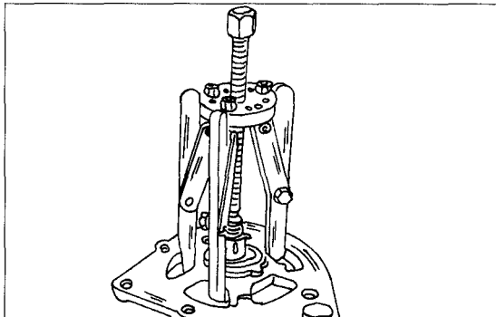
Bild 338 Abziehen des Antriebslagerschildes vom Läufer.
