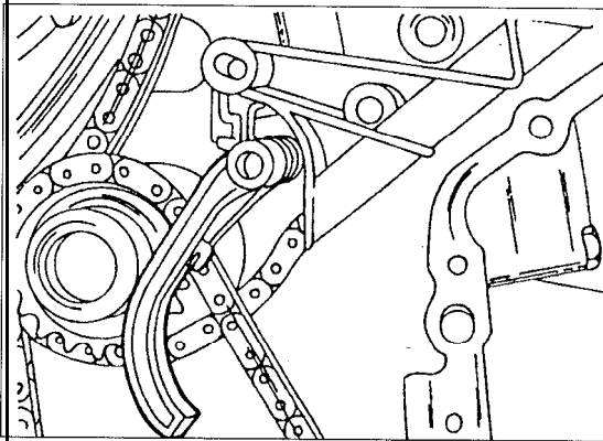
Bild 158 Spannhebel an der Kette vorbeiführen und gegen das Ende der Kurbelwelle anlegen, ehe die Gleitschiene abgezogen wird.
