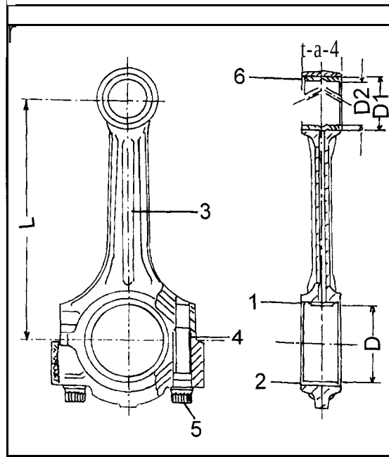
Bild 80 Schnittansicht einer zusammengebauten Pleuellstange. Die Pfeilstelle weist auf die Ölbohrung in der Pleuelaugenbüchse.
