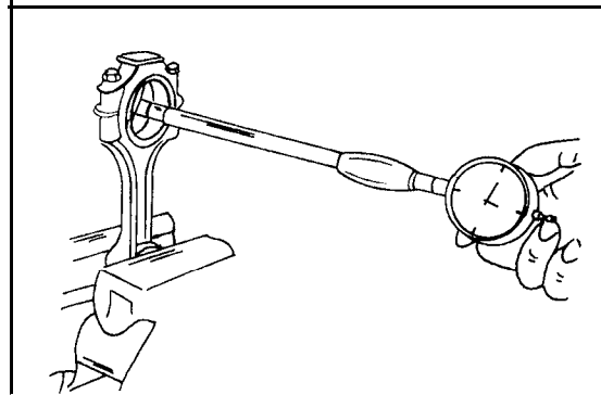
Bild 79 Ausmessen des Durchmessers der Pleuellagerschalen. Den Durchmesser an verschiedenen Stellen messen.
