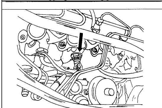
Bild 345 Lage des Gebers für die Temperatur/Vorglühanzeige beim Dieselmotor.
