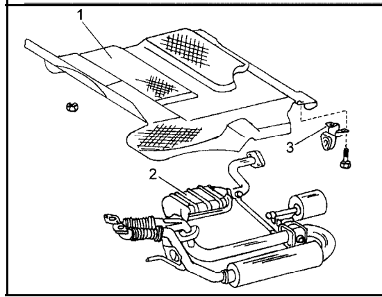
Bild 354 Zum Aus- und Einbau des Katalysators. 1 Wärmeschuttschild 2 Oxidationskatalysator 3 Aufhängungsschlaufe
