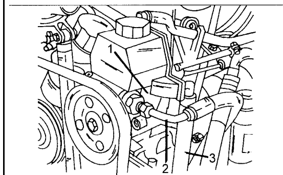
Bild 13 Ansicht des eingebauten Vorratsbehälters der Servolenkungsflüssigkeit. 1 Lenkhilfspumpe 2 Hochdruckleitung 3 Rücklaufschlauch
