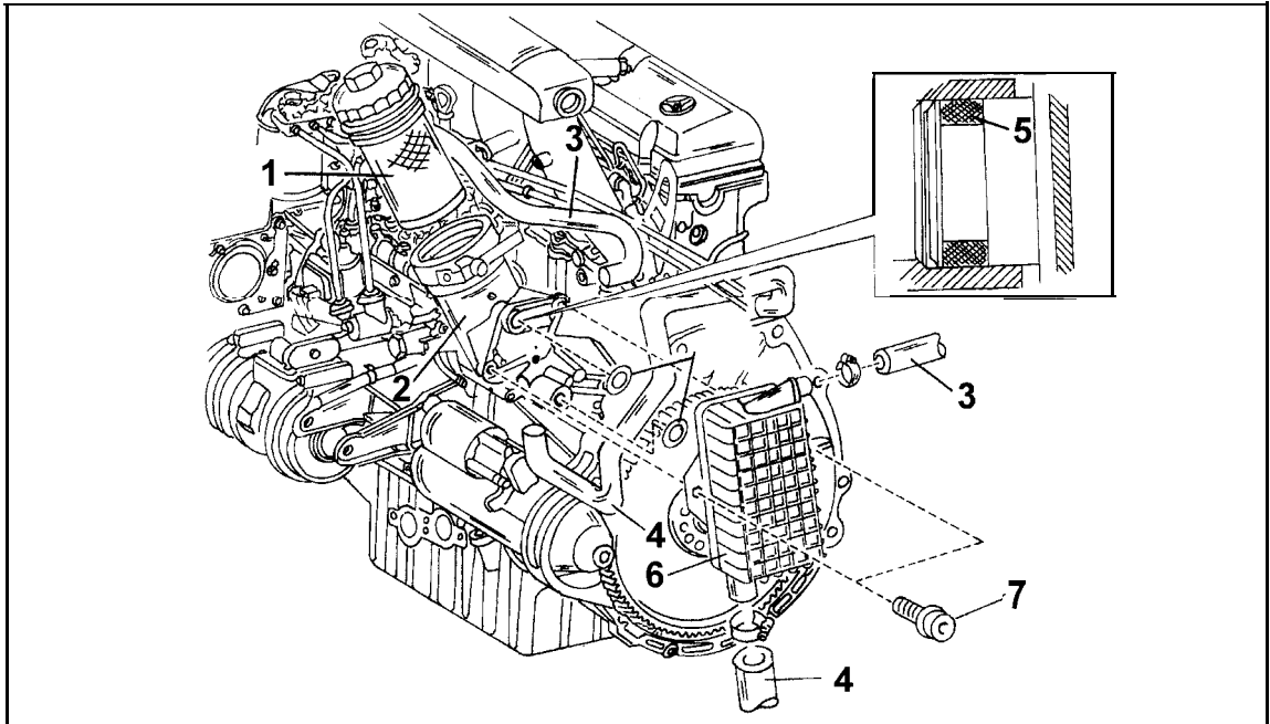
Bild 181 Einzelheiten zum Aus- und Einbau von Ölfilter und Ölkühler. 1 Ölfilter 2 Ölfiltergehäuse 3 Kühlmittelschlauch 4 Kühlmittelschlauch 5 Dichtringe 6 Ölkühler (Öl/Wasser-Wärmeaustauscher) 7 Torx-Kopf-Schraube
