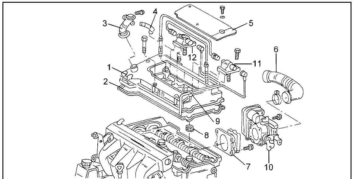
Bild 18 Einzelheiten zum Aus- und Ausbau der Zylinderkopfhaube.
