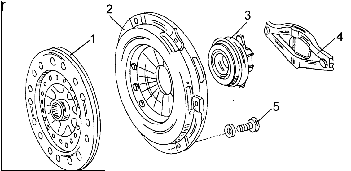
Bild 246 Die Einzelteile der Kupplung.
