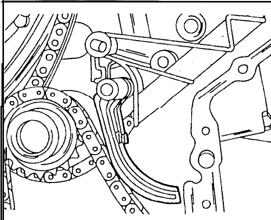
Bild 159 Der Spannhebel muss in der gezeigten Weise auf der Kette der Ölpumpe aufliegen.
