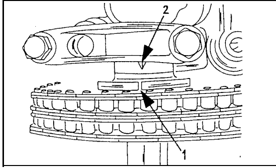
Die Stellung für den oberen Totpunkt des ersten Zylinders. Die Kerbe im Nockenwellenflansch (1) muss mit dem Ansatz am ersten Lagerdeckel der Nockenwelle (2) fluchten.
