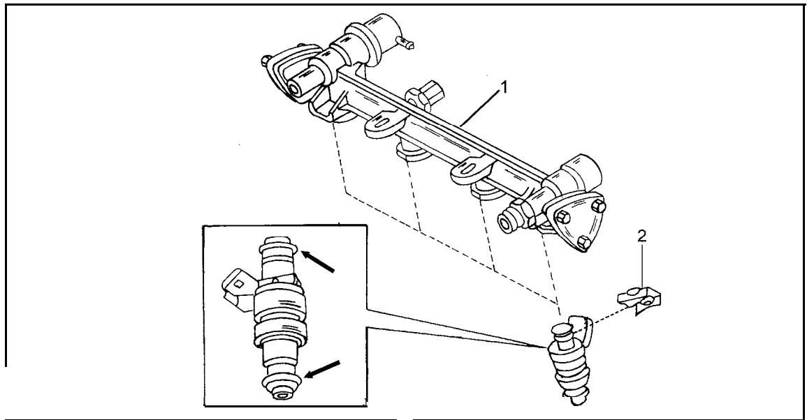
Bild 210 Einbauweise der Einspritzventile im Kraftstoffverteilerrohr. 1 Kraftstoffverteilerrohr 2 Befestigungsstück
