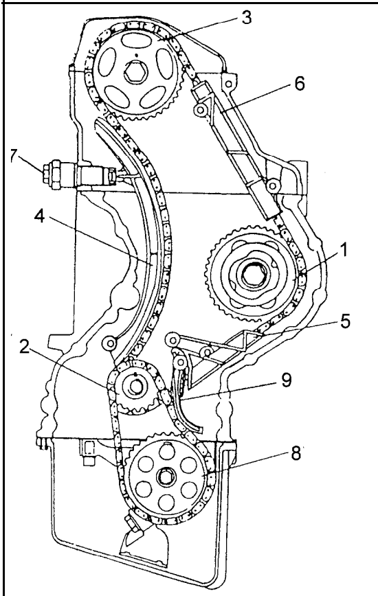
Bild 152 Ansicht der Steuerung des Motors. 1 Antrieb für Einspritzpumpe 2 Kurbelwellenkettenrad 3 Nockenwellenkettenrad 4 Spannschiene 5 Gleitschiene 6 Gleitschiene 7 Kettenspanner 8 Ölpumpenantriebsrad 9 Spannhel für Ölpumpenkette
