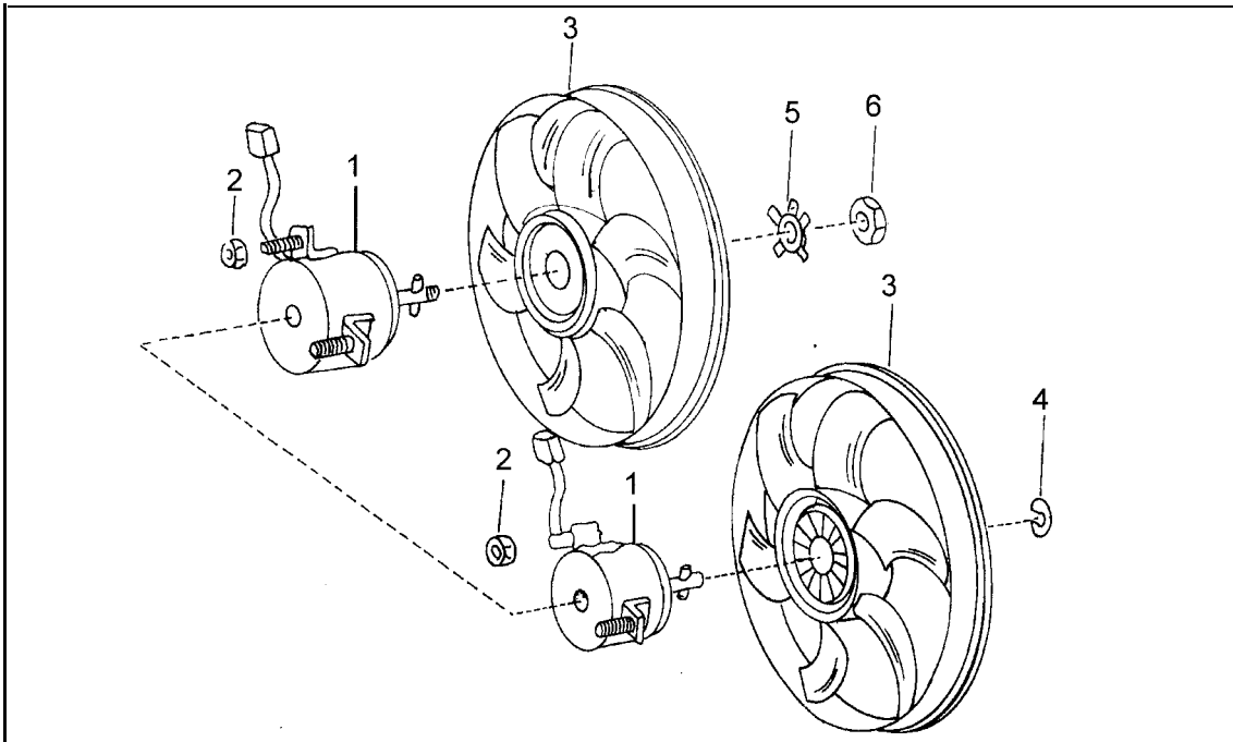
Bild 199 Die Befestigungsweise der Kühllüfter im Motorraum. 1 Lüftermotor 2 Mutter des Lüftermotors 3 Kühllüfter 4 Sicherungsspanne 5 Sicherungsblech 6 Befestigungsmutter auf Lüftermotorwelle
