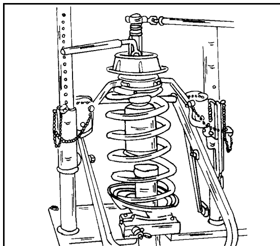
Bild 275 Vorderfedern können in der gezeigten Weise zusammengespant werden. Andere Vorrichtungen können ebenfalls benutzt werden. Die Abbildung zeigt nur einen typischen Federspanner.
