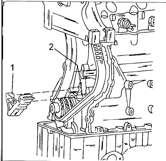
Bild 157 Die Gleitschiene (1) im Steuergehäuse wird auf den beiden Lagerbolzen (2) gehalten.
