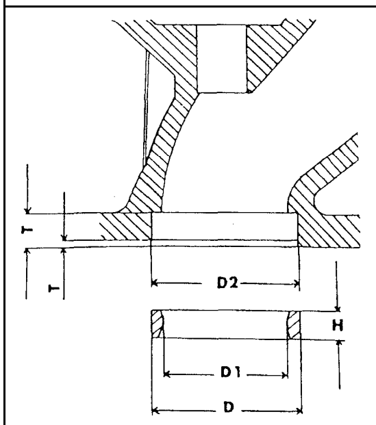
Bild 102 Die Vermessung der Ventil- sitzringe. Die Buchsta- ben haben die folgende Bedeutung:
