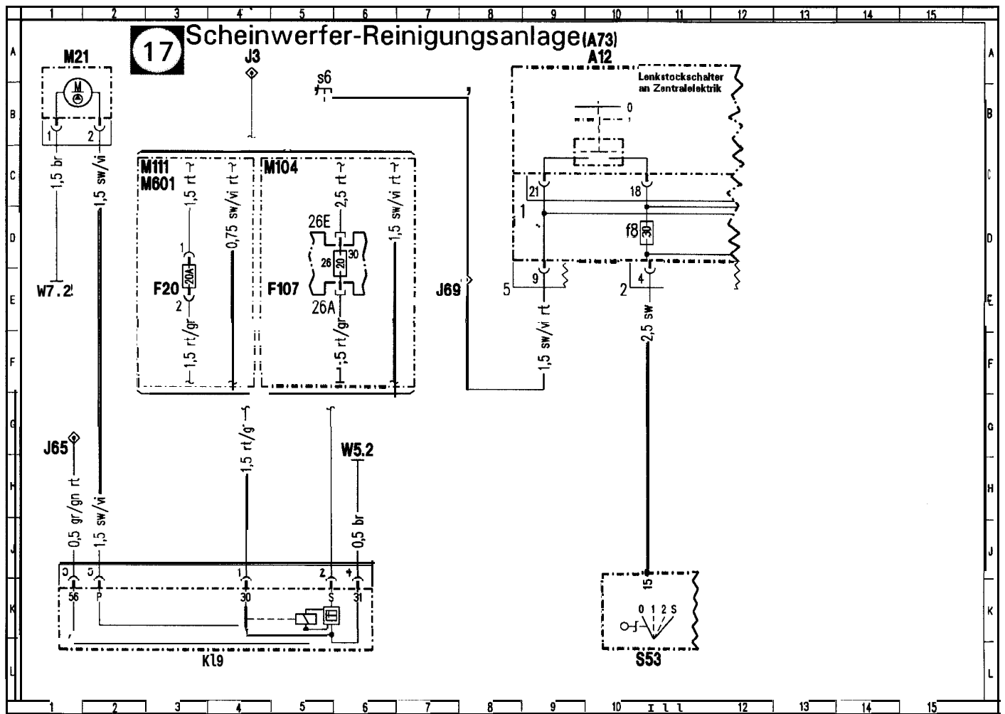
Schaltplan 17 -Scheinwerfer-Reinigungsanlage
