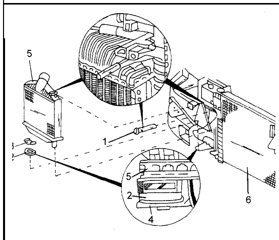
Bild 235 Einzelheiten um Aus- und Einbau des Ladeluftkühlers.
