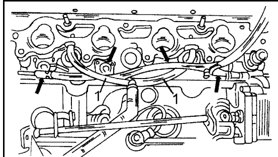
Bild 24 Die Unterdruckleitungen (1) an der Seite des Zylinderkopfes abschliessen und die mit den Pfeilen gezeigten Stecker abziehen
