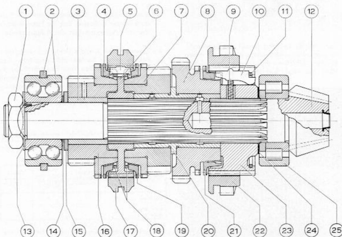
Triebbling — Schnittbild
