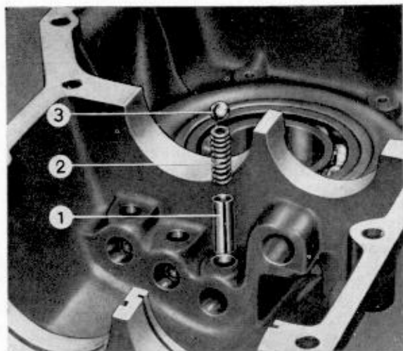
1 - Führungshülse 2 - Feder 3 - Riegelkugel
