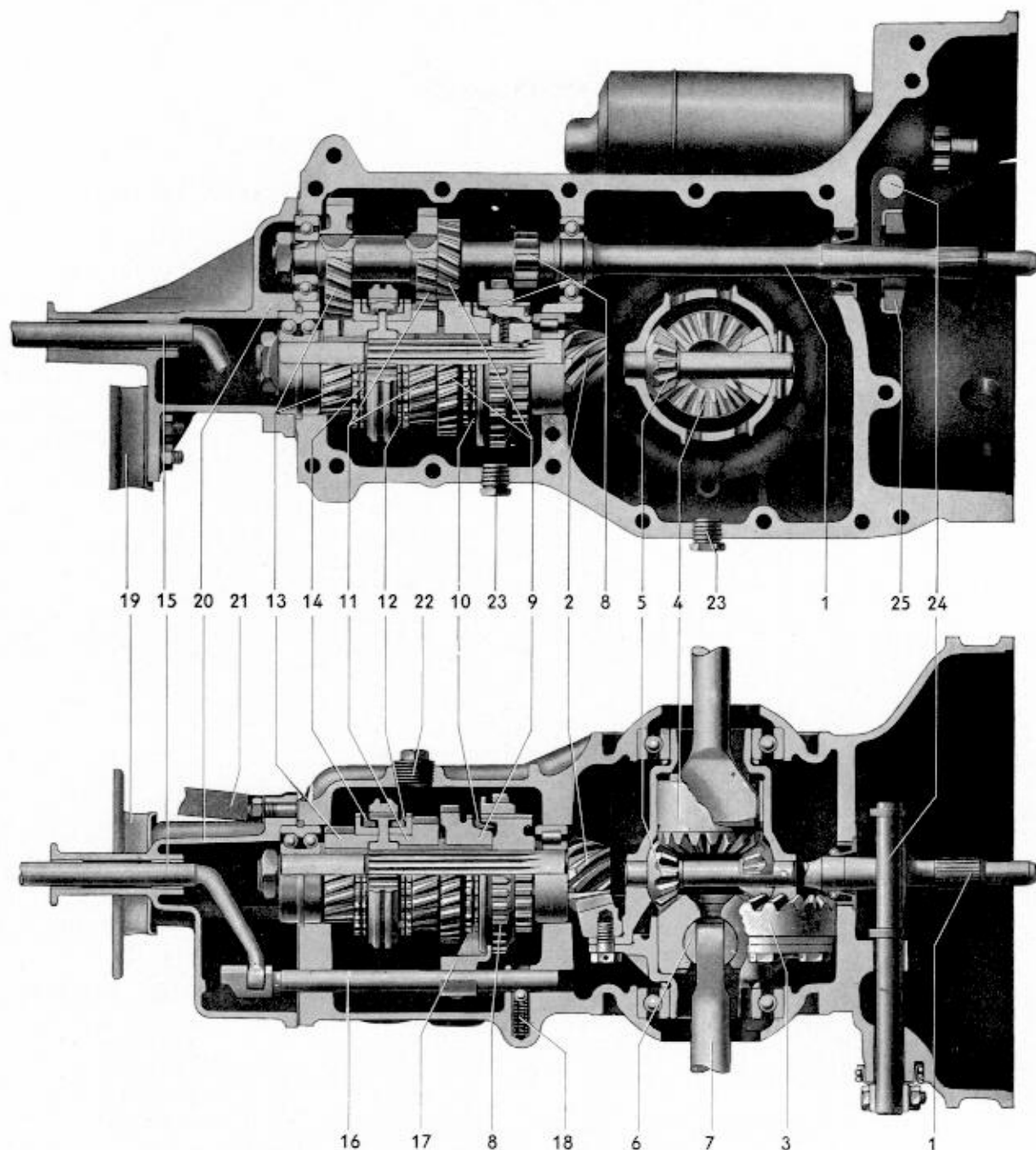
Volkswagen — Hinterachse und Getriebe (Schnittbild)
