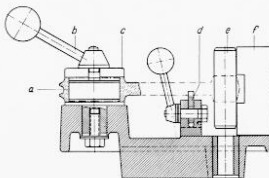
Vorrichtung 214
