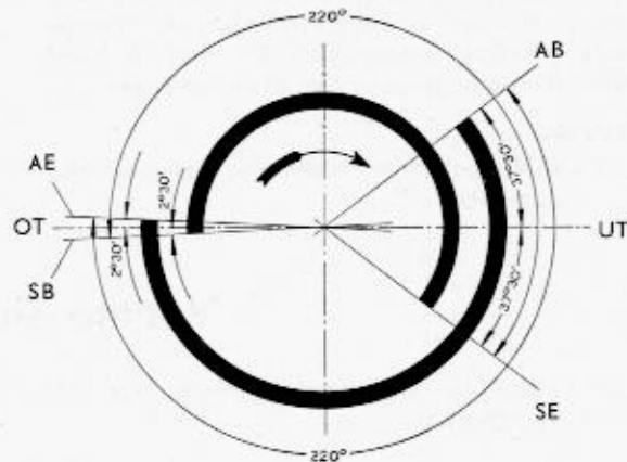
Steuerzeiten
