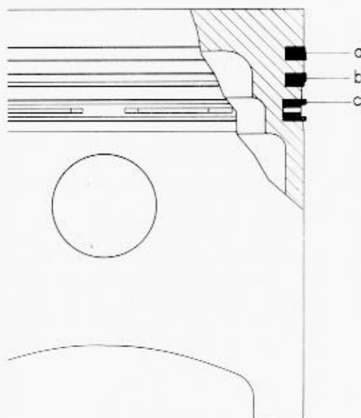
a - Topring b - Nasenkolbenring c - Ölabbstreifring
